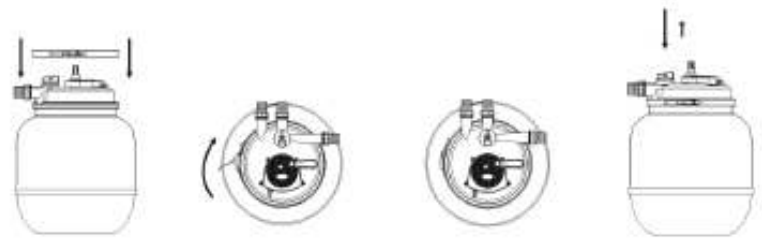
Lukning af filter med placering af spændering / Placering spänning vid låsning av filter
